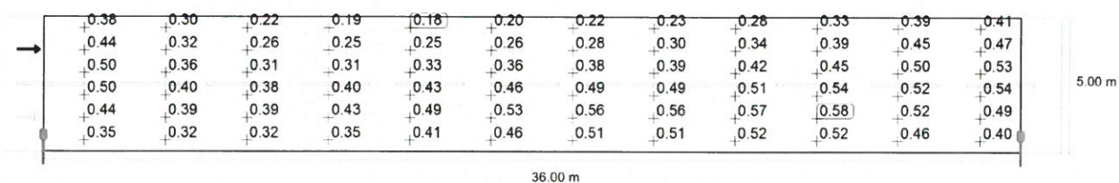
Observator 2: Valoarea de întreținere, densitatea luminii cu carosabil uscat [ \text{cd/m}^2 ] (Raster valoric)
