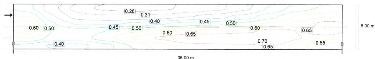
Observator 2: Densitatea luminii la instalația nouă [ \text{cd/m}^2 ] (Linii Isolux)
